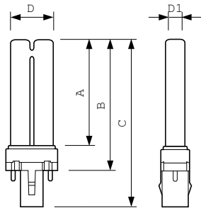
TUV 9W PL-S
